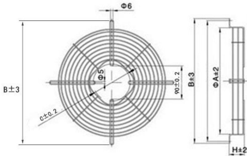
电机风叶网罩安装图
